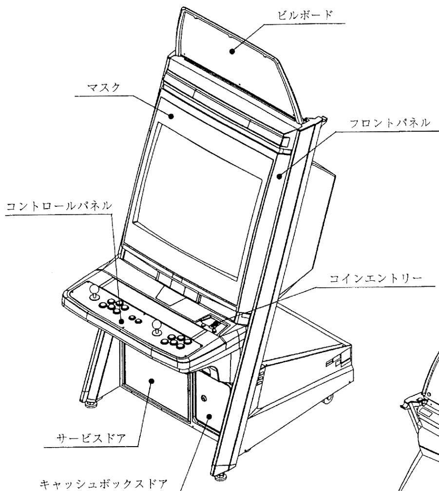
図4 a 全体図
