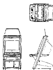
図6. 1d 1/100の図です。設置場所へのレイアウトの参考にしてください。
